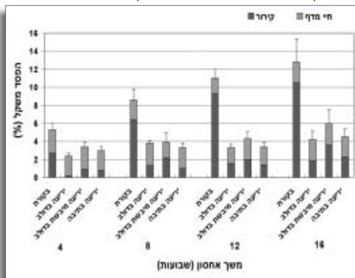
איור 2: השפעת עטיפה בשקיות Xtend® שונות על הפסד המשקל של פירות רימון מזן 'וונדרפול' לאחר הקטיף. המדידות נערכו כעבור פרקי זמן שונים של ארבעה, שמונה, 12 ו-16 שבועות אחסון (עמודה כהה) וחמישה ימים נוספים של שהייה בתנאים של חיי מדף ב-20 מ"צ (עמודה בהירה). התוצאות הן ממוצעים ± ש.ת. של עשר חזרות
